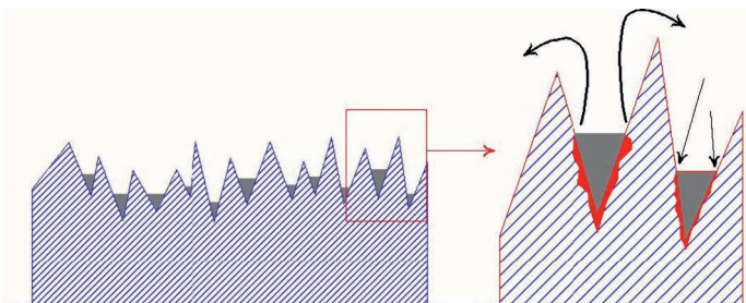
Afbeelding 7 Geslepen en/of ruw oppervlak dat schematisch sterk uitver-groot is. Vuil en andere depositiën zorgen ervoor dat chloriden diep door-dringen onder deze afzettingen waardoor het oppervlak ter plaatse aange-tast wordt. Corrosieproducten zoals dan uitreden in de vorm van pokken bij aluminium.
